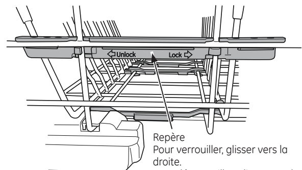
Attache de barre
