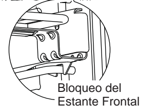
Sostenga el riel frontal superior y las manijas inferiores y empuje el estante hasta que la función de instalación se bloquee en el soporte frontal.
