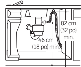
Installation avec broyeur à déchets
