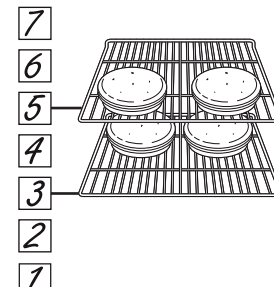
Position de la grille pour Cuisson à Convection, les gâteaux à l'arrière de la grille 3 et à l'avant de la grille 5.
