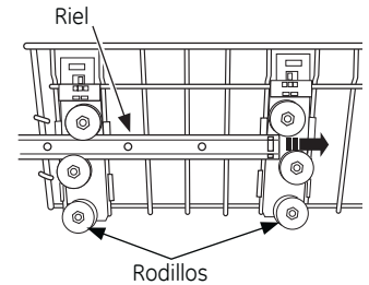
Rodillos
